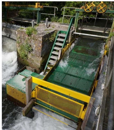
Figure 8 : Vue du dispositif de piégeage de dévalaison d'Eu
